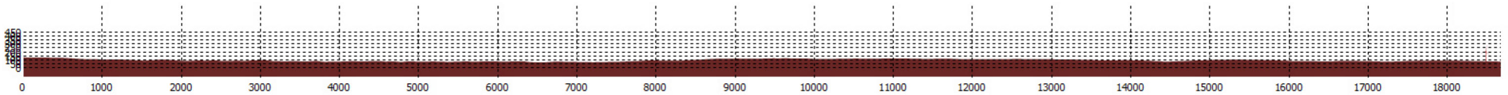
Coupe topographique vers E3 avec échelle proportionnelle verticale / horizontale.
